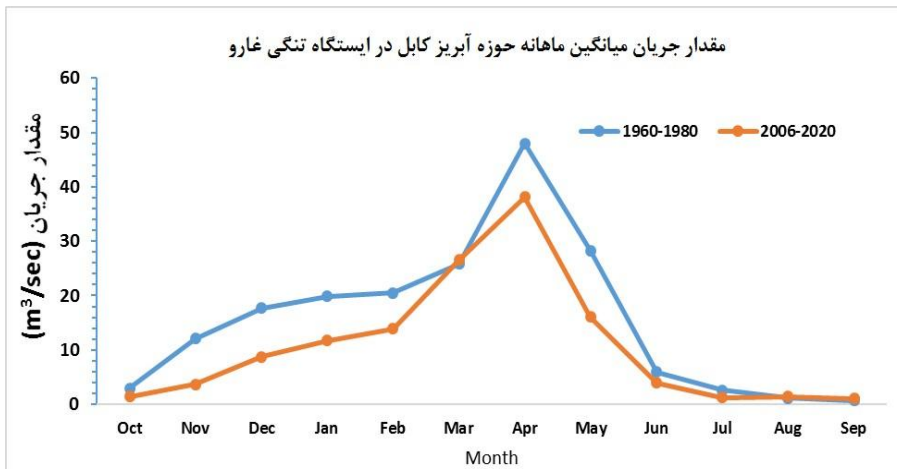
شکل (۴): نمودار مقایسه مقدار جریان میانگین جدید و تاریخی در ایستگاه تنگی‌غارو حوضه آبریز کابل.
