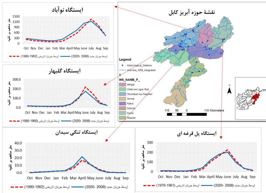
شکل (۵): موقعیت جغرافیایی و نمودار مقایسه مقدار جریان میانگین جدید و تاریخی در چهار ایستگاه حوضه آبریز کابل.
