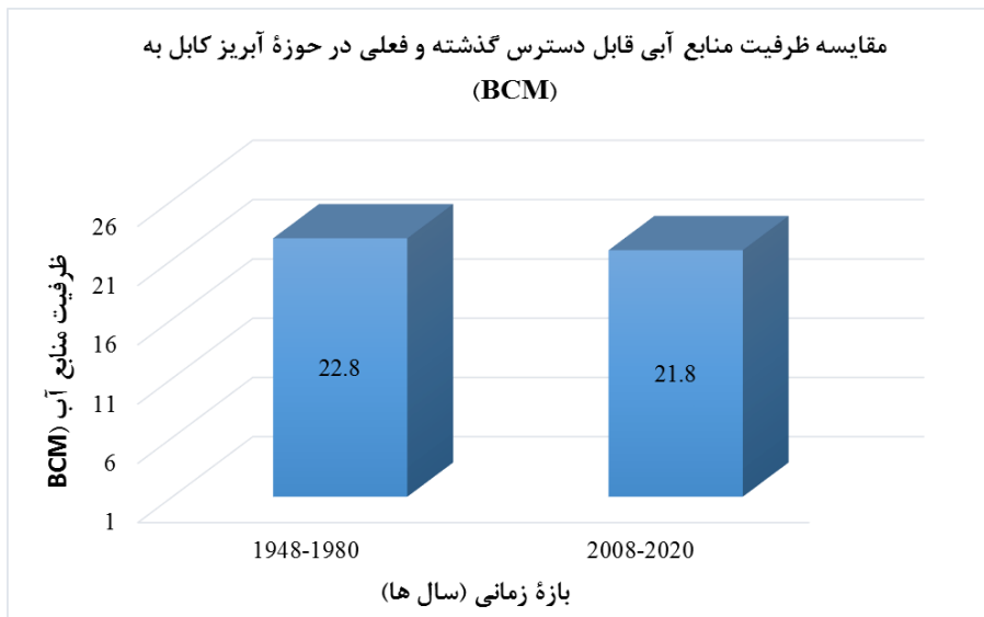
شکل (۶): مقایسه ظرفیت منابع آب قابل دسترس در دو بازه زمانی ۱۹۴۸-۱۹۸۰ و ۲۰۰۸-۲۰۲۰
