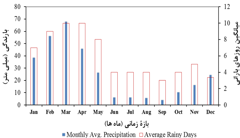
شکل (۳): میانگین بارش ماهانه درازمدت و روزهای بارانی حوضه کابل بازه زمانی ۱۹۷۹-۲۰۲۰.
